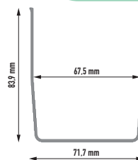
Przekrój rynny
