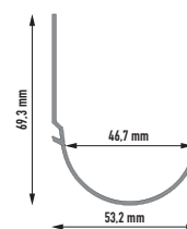
Przekrój rynny
